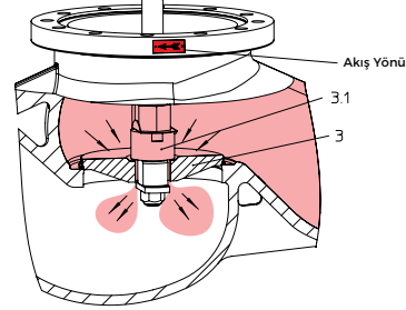
Dengeleme klapele gövde kesiti.
